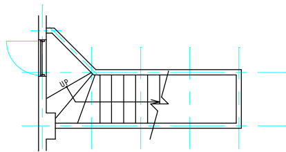
1階平面図
